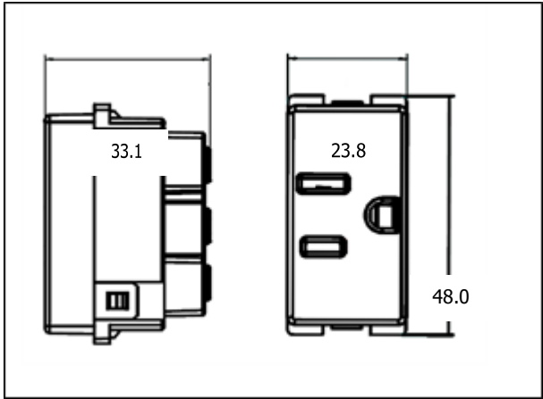
Figura 4. Receptáculo sencillo
